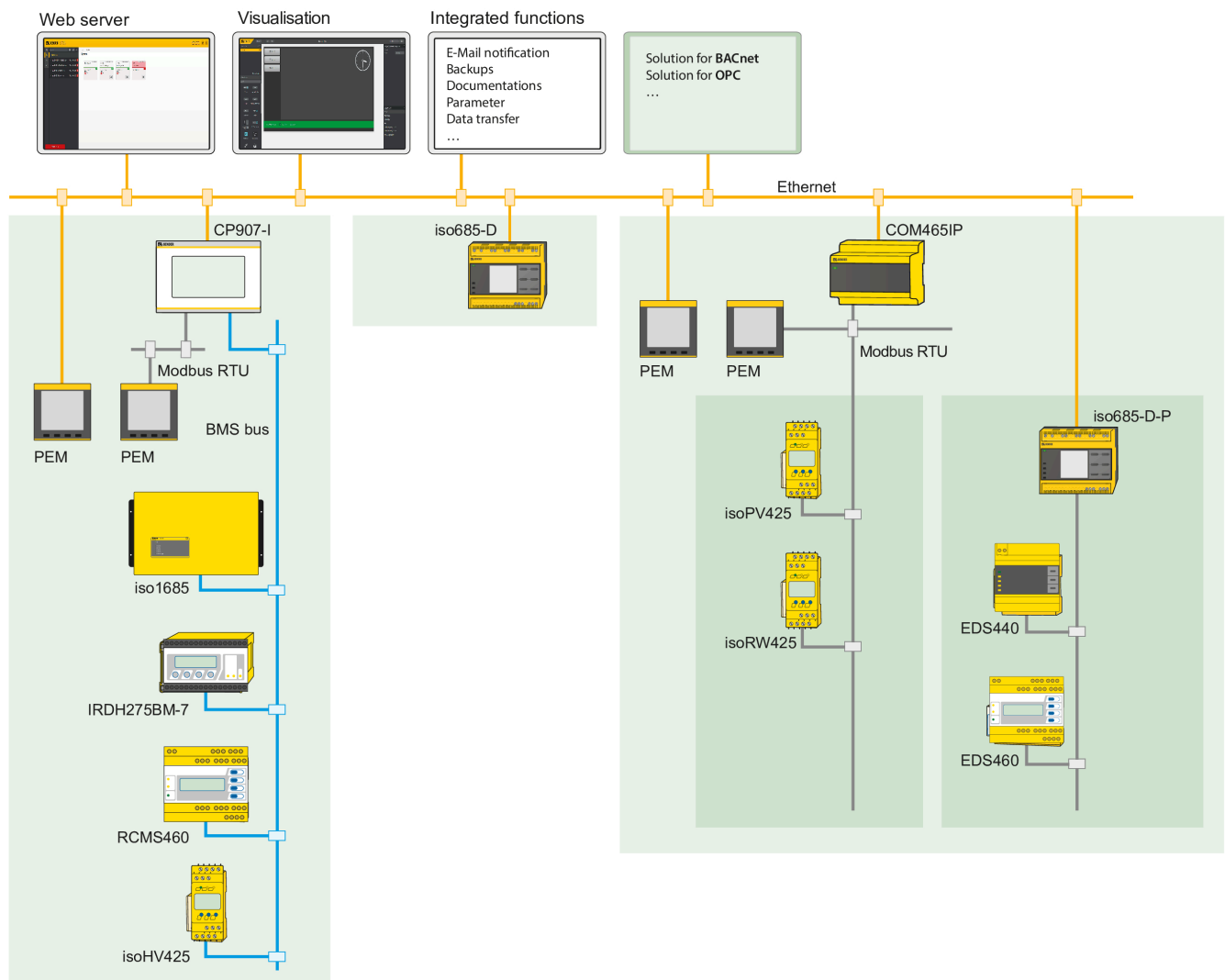
Schematic diagram COM465...P
